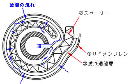
モジュール断面図
