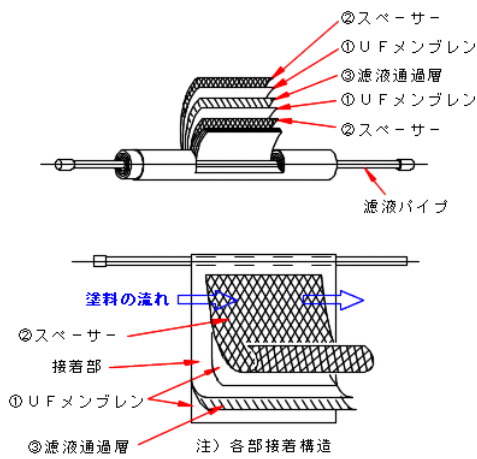
モジュール断面図
